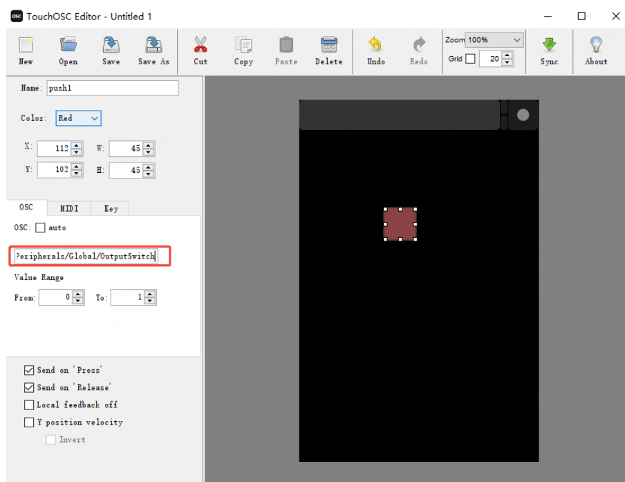
Figure 6-9 OSC parameter settings
